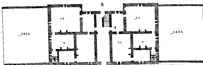
PRIMA ICHNOGRAPHIA PRIMAE CONTIGNATIONIS
