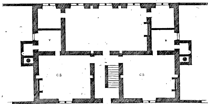
ICHOGRAPHIA
