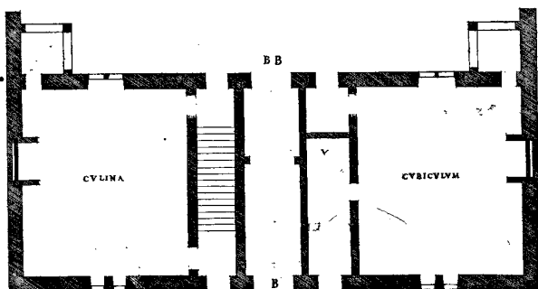
PRIMA ICHNOGRAPHIA PRIMÆ CONTIGNATIONIS
