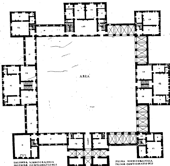
SECONDA ICHNOGRAPHIA SECONDAE CONTIGNATIONIS
