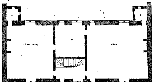
SECUNDA ICHNOGRAPHIA SECUNDA CONTIGNATIONIS
