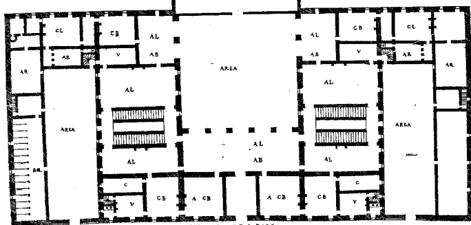
ICHOGRAPHIA
