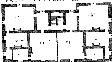
TERTIA ICHNOGRAPHIA TERTIAE CONTIGNATIONIS
